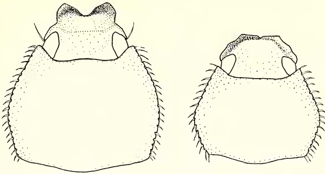
Abb. 1: Kopf und Pronotum von Maechidius lobaticeps n. sp. (links ♂, rechts ♀)
